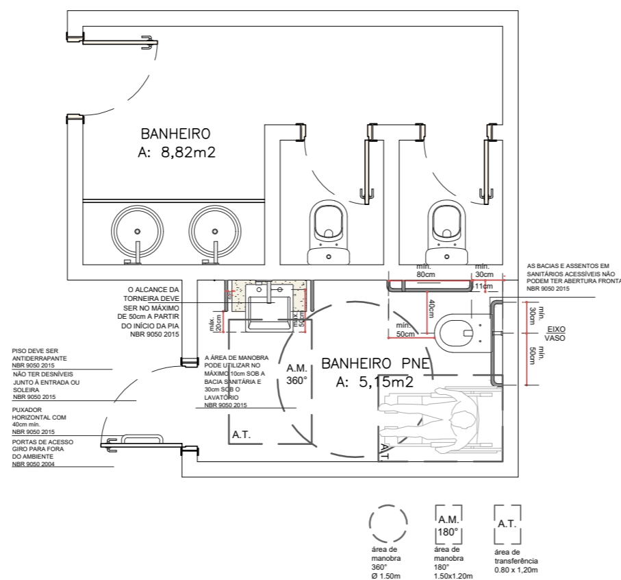
Banheiro existente 02 - Reforma e ampliação PNE ESC. 1:50
