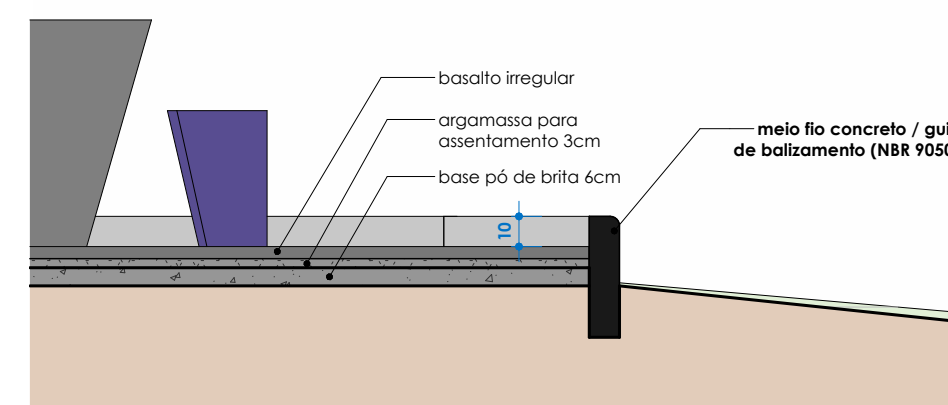
Det 1 / Acessibilidade ESC: 1 : 25
