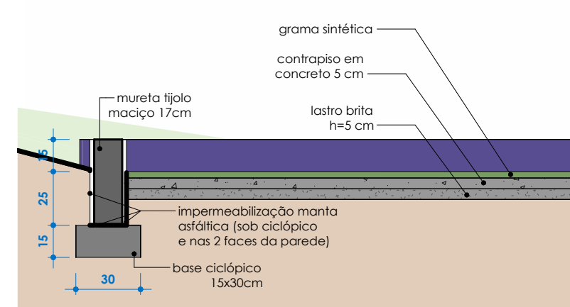
Det 2 / Piso grama sintética ESC: 1 : 25
