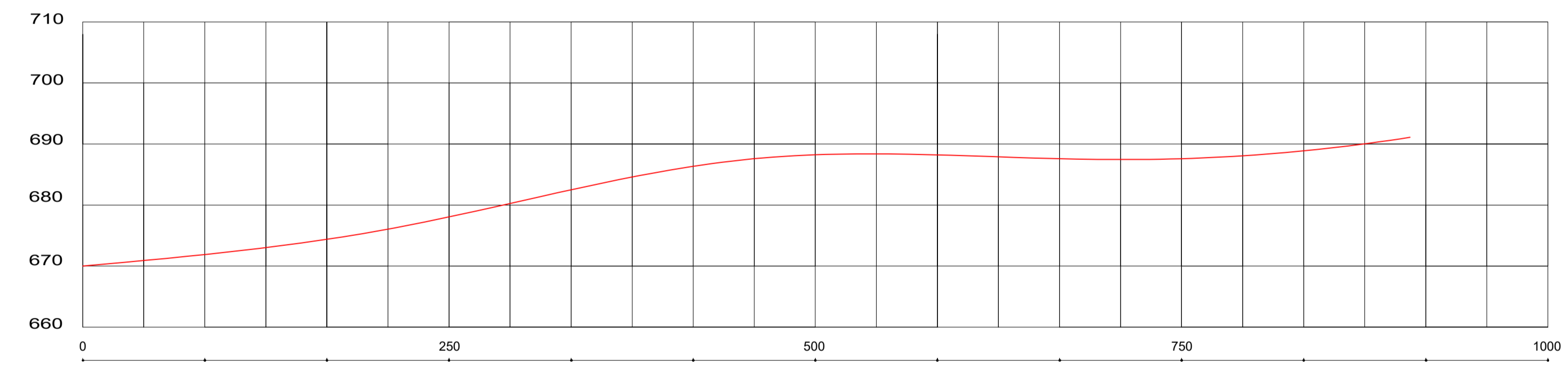
PERFIL DE ELEVAÇÃO DO TRECHO PARA CAPEAMENTO DA AV. BARROS CASSAL
