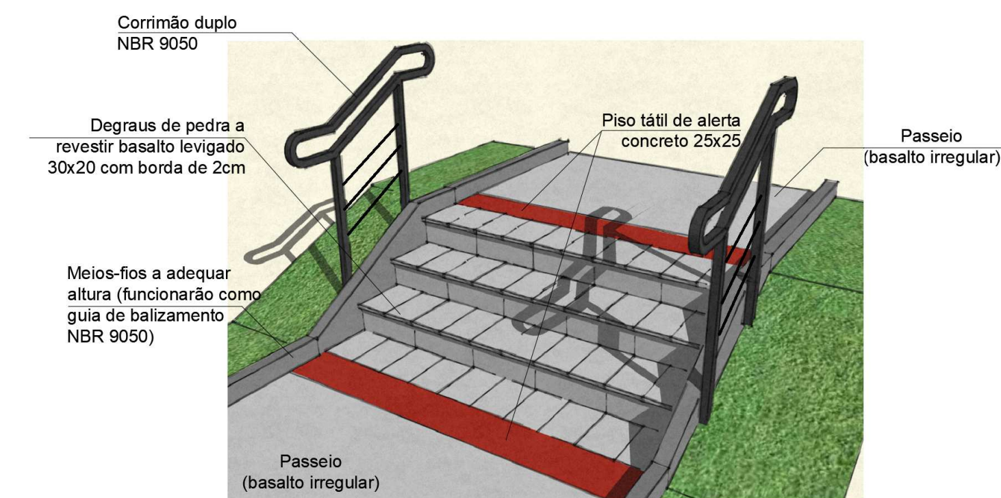
De1 - Guardacorpas e revestimento degraus ESC: 1 : 25
