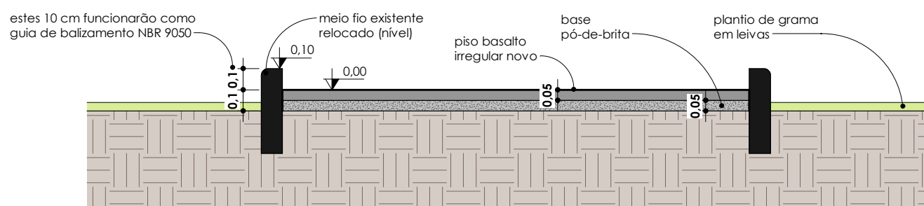
De12 - Perfil das caçadas novas ESC: 1 : 25
