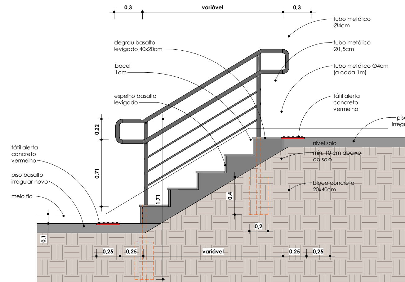
De1 - Guardacorpas e revestimento degraus ESC: 1 : 25
