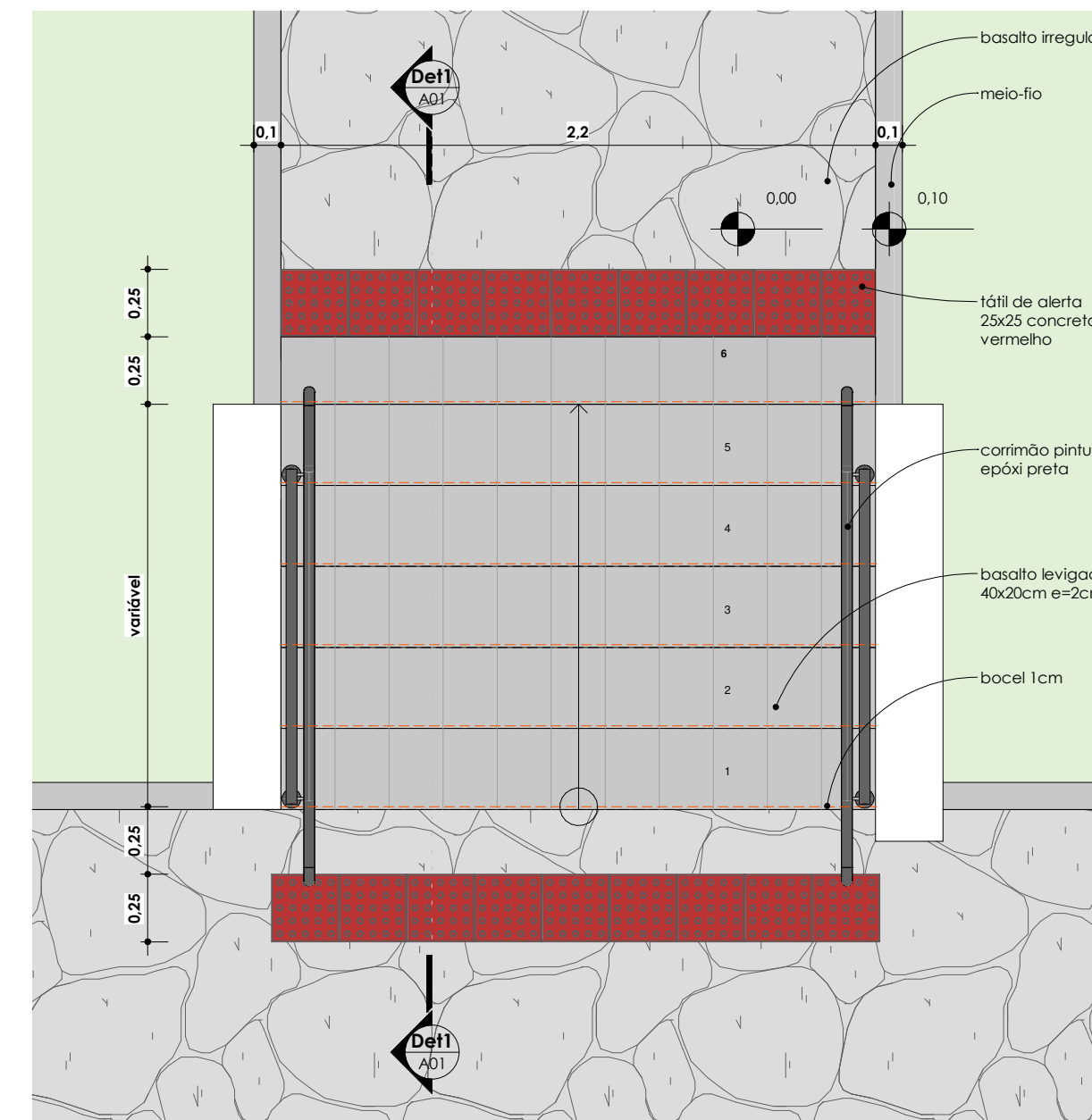
Detalhe escadas ESC: 1 : 25
